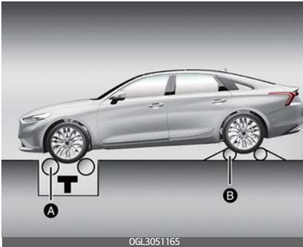
[A] 속도계 검사 롤 테스터
